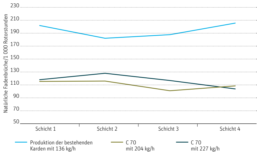
Abb. 2: Das Band der optimierten Karde C 70 zeigt auch mit hoher Produktion ein sehr gutes Laufverhalten auf der Rotorspinnmaschine.
